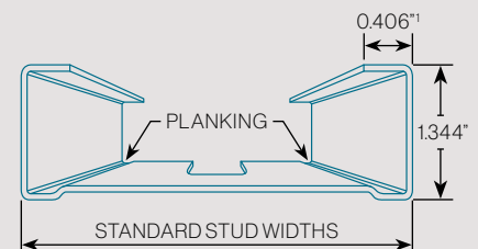
PrimeWall® 20 EQ Stud
